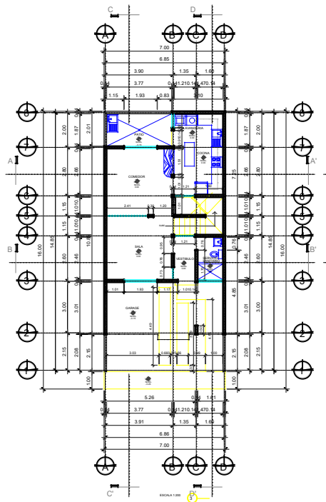
PLANTA ACOTADA
